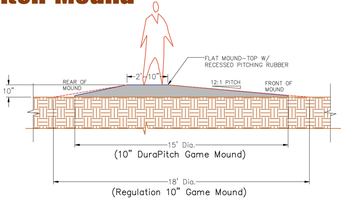
LONGITUDINAL SECTION
